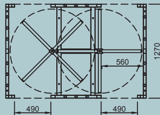
A-A KESİT
